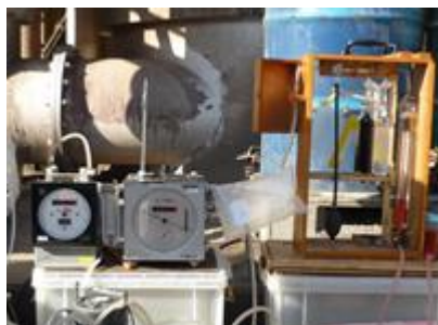
排ガス物質のモニタリング、および測定を行う装置。
