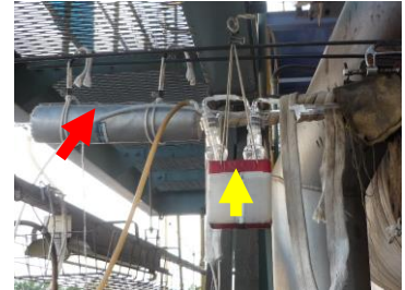
奥の灰色の筒状の機器(赤印)でダイオキシンを、手前のガラス機器(黄印)で塩化水素を測定しています。
